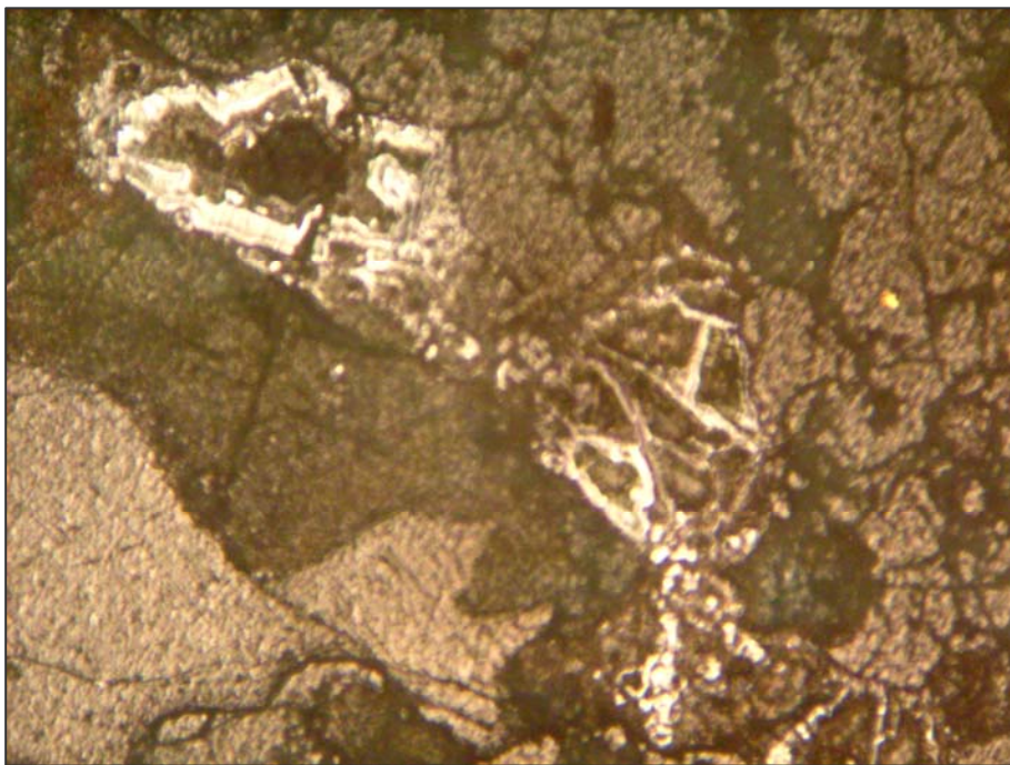
شکل (۳-۱۴): تصویری از مقطع صیقلی نمونه شماره F-258
