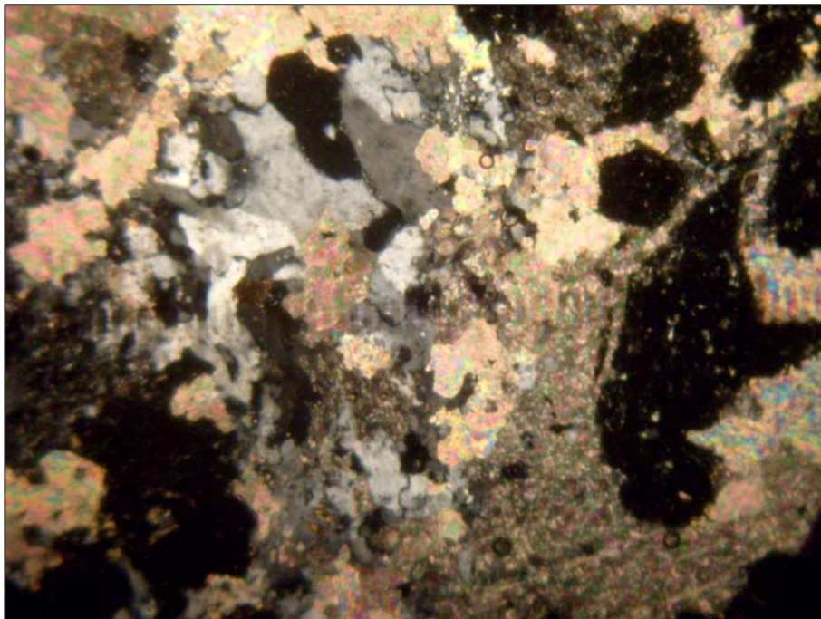
شکل (۸-۳) : تصویری از مقطع نازک نمونه شماره F-255 در نور XPL
