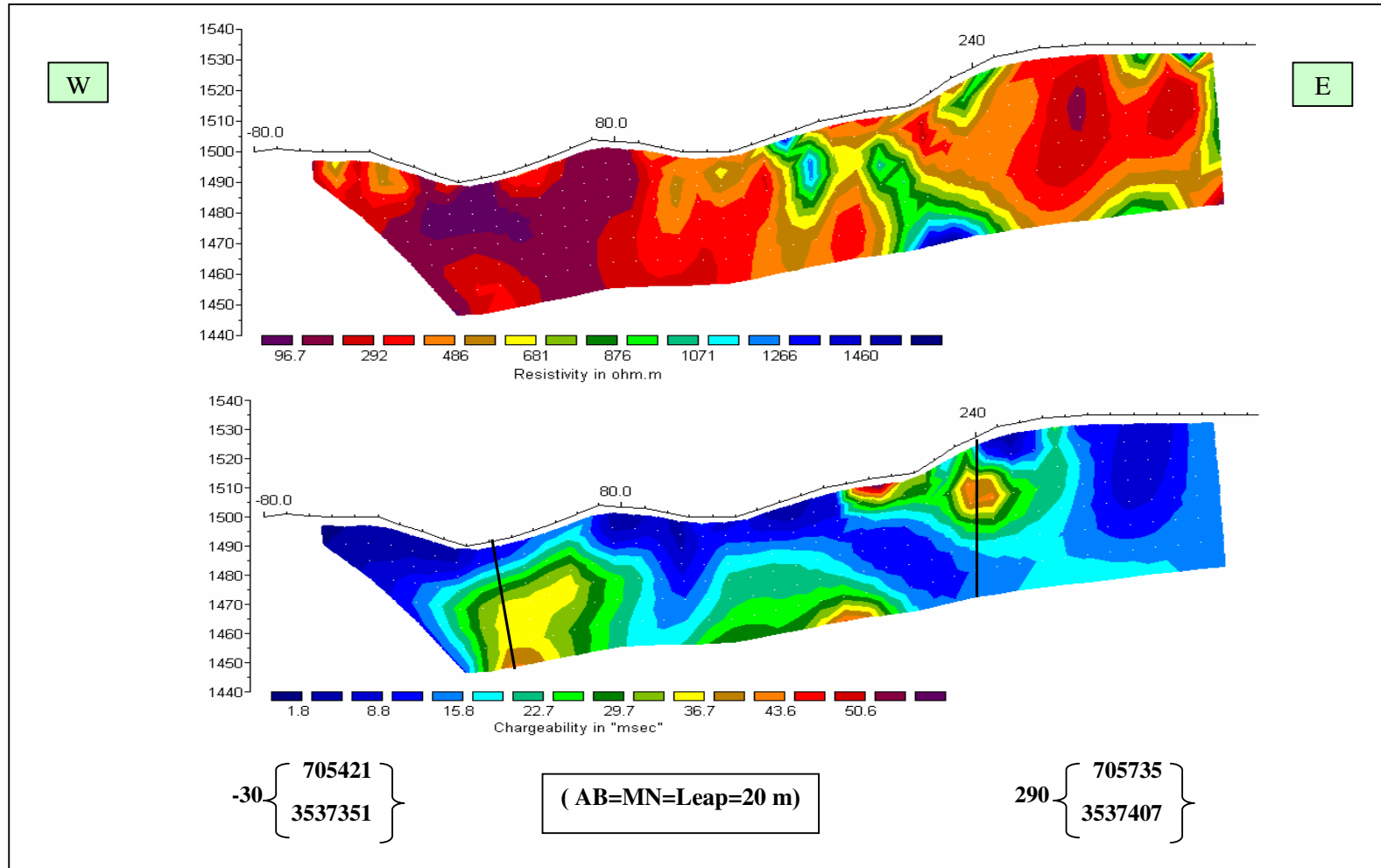
نقشه شماره ۳۷: مدل مقاومت ویژه ظاهری و پلاریزاسیون القایی دایبل دایبل شماره ۶ روی پروفیل 400N
