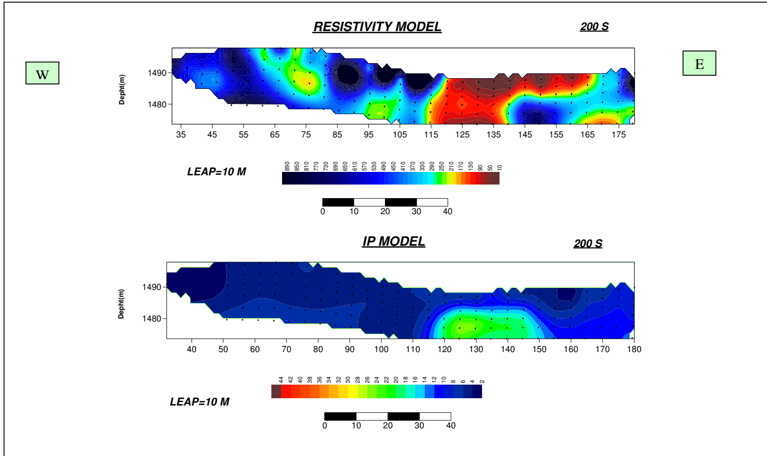
نقشه شماره ۱۲: مدل مقاومت ویژه ظاهری و پلاریزاسیون القایی دایپل دایپل شماره ۱ روی پروفیل 200S(10meter) در محیط surf
