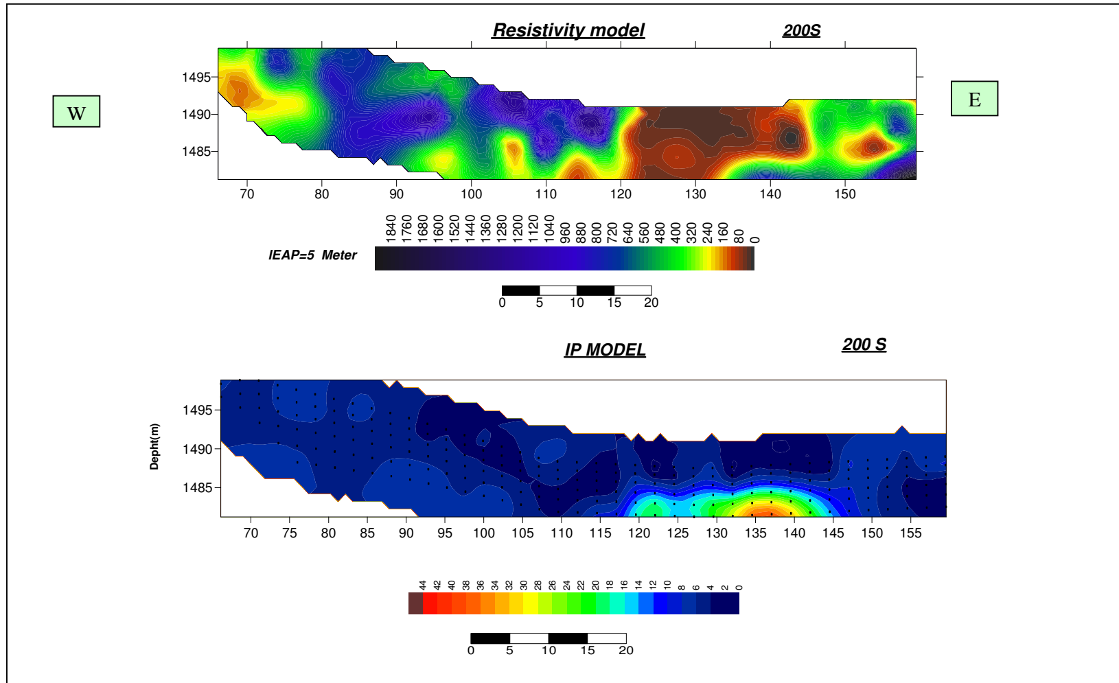
نقشه شماره ۸: مدل مقاومت ویژه ظاهری و پلاریزاسیون القایی دایپل دایپل شماره ۱ روی پروفیل 200S(5meter) در محیط surfer
