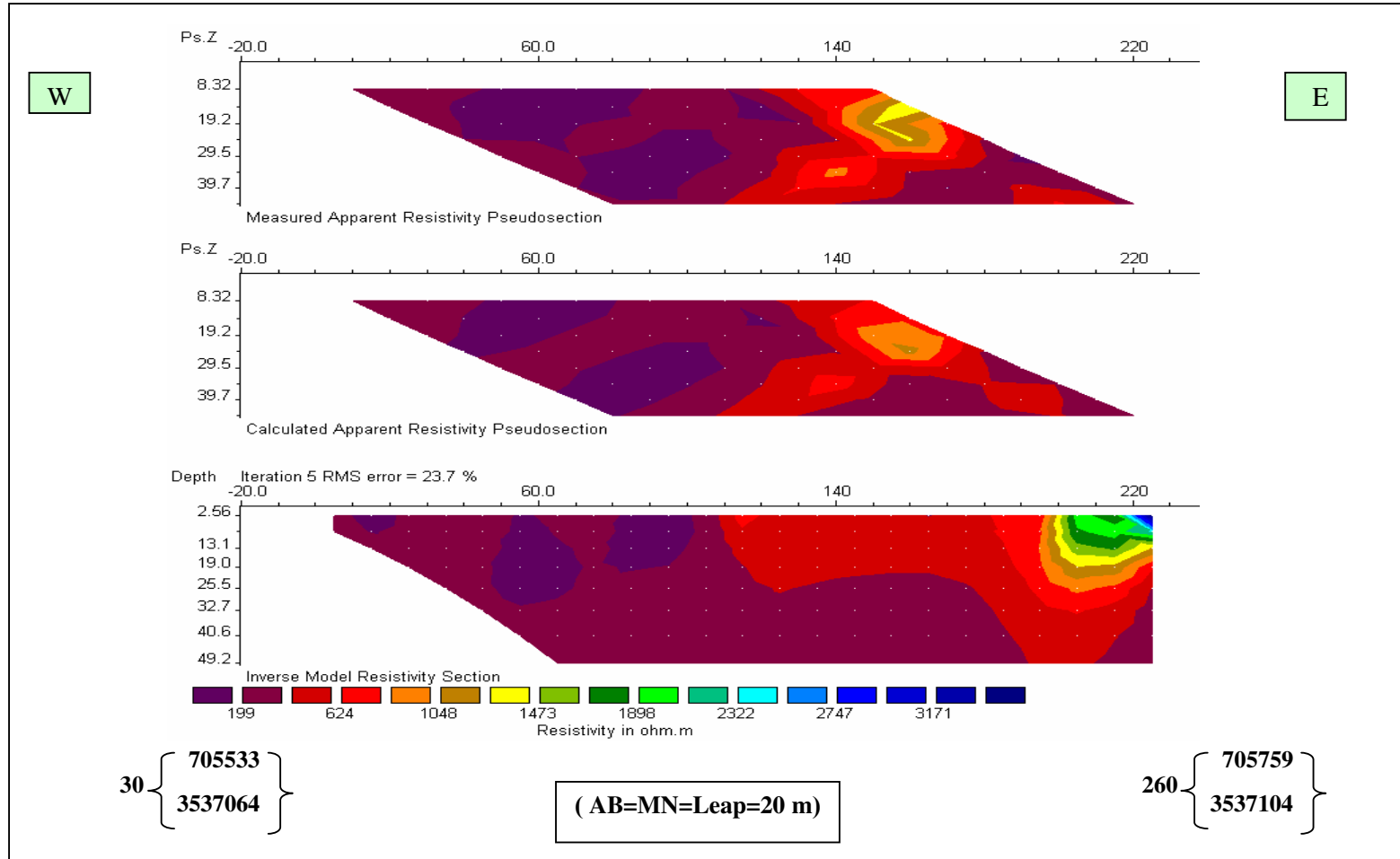
نقشه شماره ۲۶: شبه مقطع مقاومت ویژه ظاهری به همراه مدل دایبل دایبل شماره ۳ روی پروفیل 100 N
