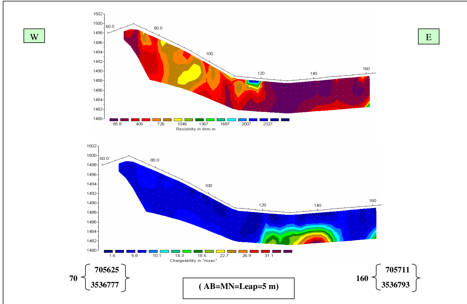
نقشه شماره ۵: مدل مقاومت ویژه ظاهری و پلاریزاسیون القایی دایبل دایبل شماره ۱ روی پروفیل (200 S (5meter)
