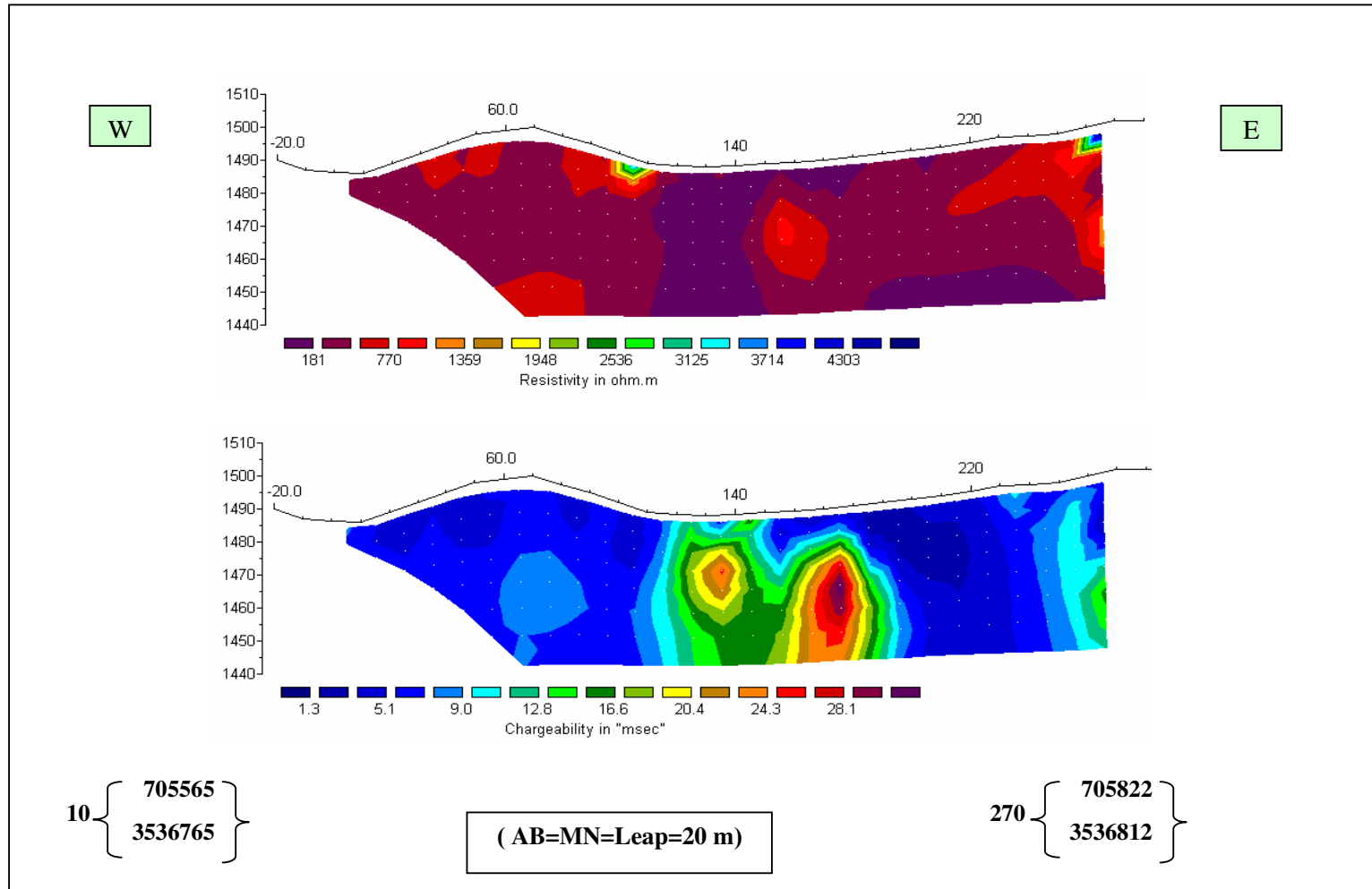
نقشه شماره ۱۳: مدل مقاومت ویژه ظاهری و پلاریزاسیون القایی دایبل دایبل شماره ۱ روی پروفیل 200 S
