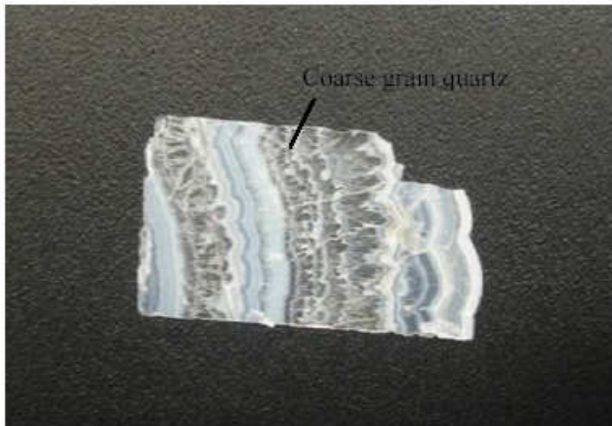
شکل ۱: تصویری از نوارهای دانه درشت و دانه ریز در رگه های کوارتزی منطقه
