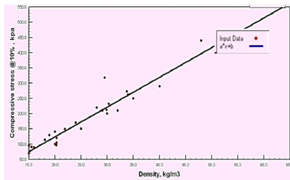
شکل ۶ نمودار تنش فشاری در ۱۰ درصد تغییر شکل در برابر چگالی EPS
