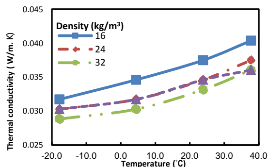
شکل ۳ نمودار ضریب هدایت حرارتی EPS در برابر دما در چگالی‌های مختلف [۳]
