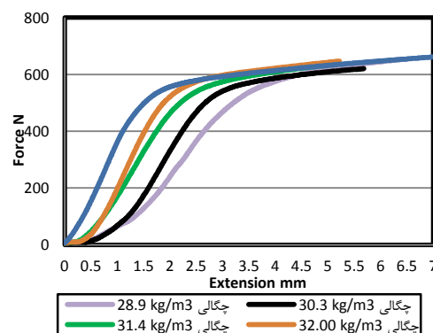
شکل ۵ نمودار نیرو - تغییر شکل نمونه های EPS با چگالی زیاد
