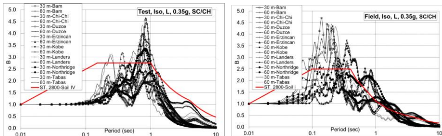
الف) ستون ۳۰ متری خاک نوع I، مینا سرعت موج برشی صحرائی ب) ستون ۳۰ متری خاک نوع IV، مینا سرعت موج برشی آزمایشگاهی
