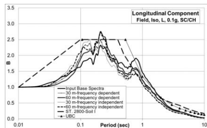
الف) خاک نوع I، مبنا سرعت موج برشی صحرائی
