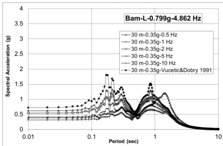
الف) ستون ۳۰ متری خاک نوع I، مبنا سرعت موج برشی صحرائی ب) ستون ۳۰ متری خاک نوع IV، مبنا سرعت موج برشی آزمایشگاهی شکل ۶. طیف‌های پاسخ شتاب مؤلفه L زلزله بم (PGA=0.35g) با استفاده از منحنی‌های رفتاری متأثر از اثر فرکانس
