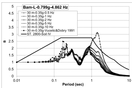
الف) ستون ۳۰ متری خاک نوع I، مبنا سرعت موج برشی صحرائی ب) ستون ۳۰ متری خاک نوع IV، مبنا سرعت موج برشی آزمایشگاهی شکل ۷. مقایسه ضریب شکل طیف مؤلفه L زلزله بم (PGA=0.35g) حاصل از کاربرد منحنی‌های رفتاری متأثر از اثر فرکانس با ضریب شکل طیف طرح استاندارد ۲۸۰۰
