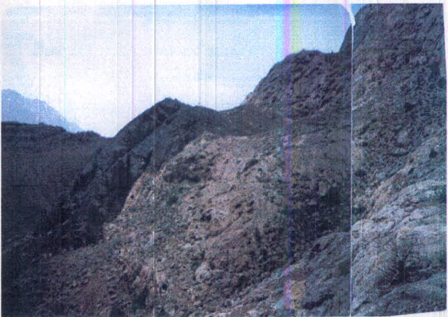
شکل ۴-۱۲ بانورامایی از وضعیت کنتاکت آهکهای الیکا ، سیلهای بازیک تا حد واسط و شیلهای شمشک در کوه بیش سر و امتداد ۲۳۰ درجه
