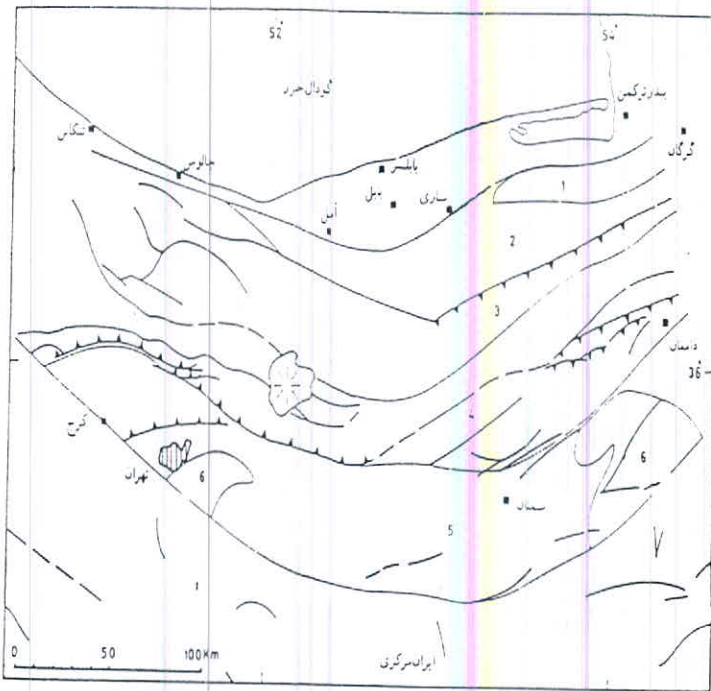
شکل ۳-۳ تقسیمات زون های ساختمانی البرز مرکزی بر مبنای گسل ها و رورانگی های بزرگ (اشتوکلین ، ۱۹۷۴)
