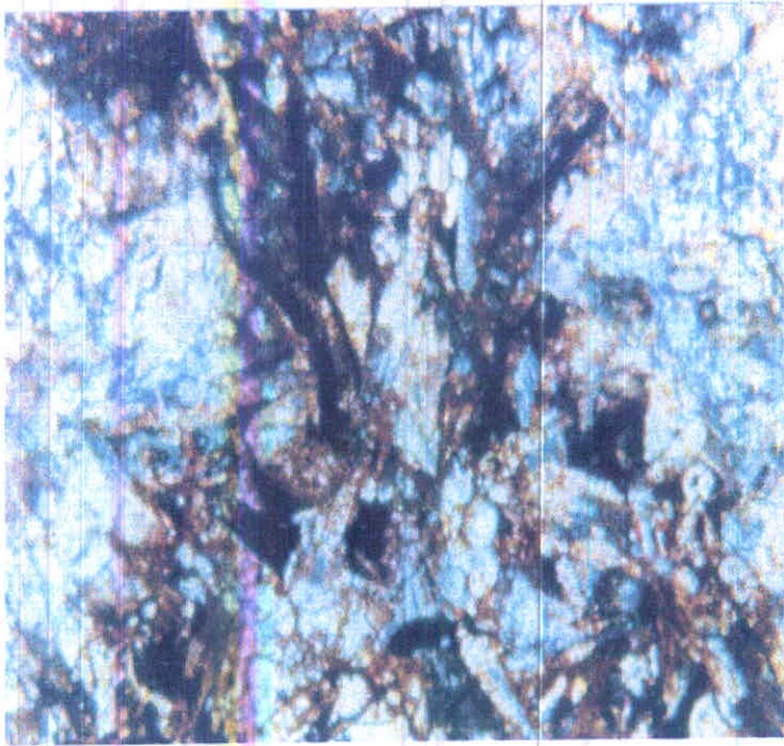
شکل ۴-۴ عکس مریوگراف به مقطع نمونه شماره ۱۷
