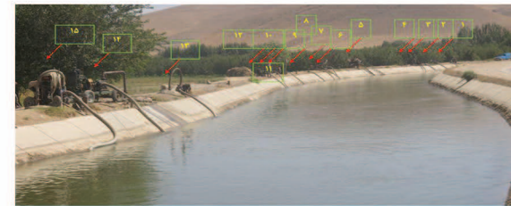
شکل ۲- وضعیت برداشت از کانال آب زربینه رود توسط موتور و تلمبه‌ها
