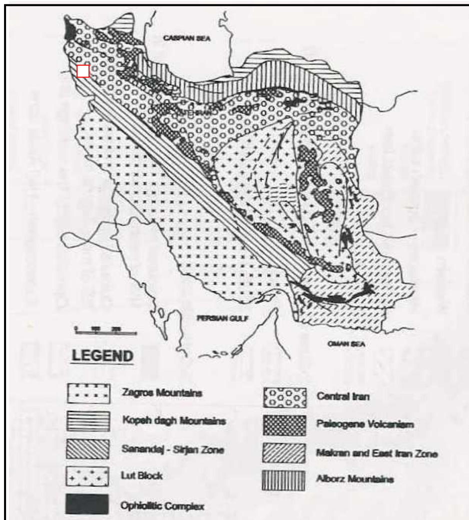
شکل ۳) زون های ساختاری - رسوبی ایران (بر اساس اشتوکلین، ۱۹۶۸) و موقعیت منطقه اکتشافی در آن. منطقه مورد مطالعه بخشی از زون دگرگونی سنندج - سیرجان است.
