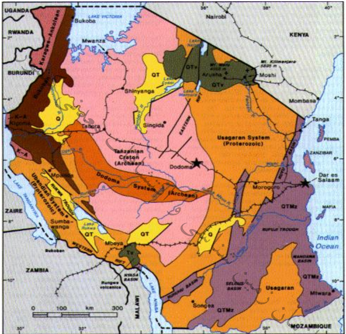
نقشه زمین شناسی کشور تانزانیا
