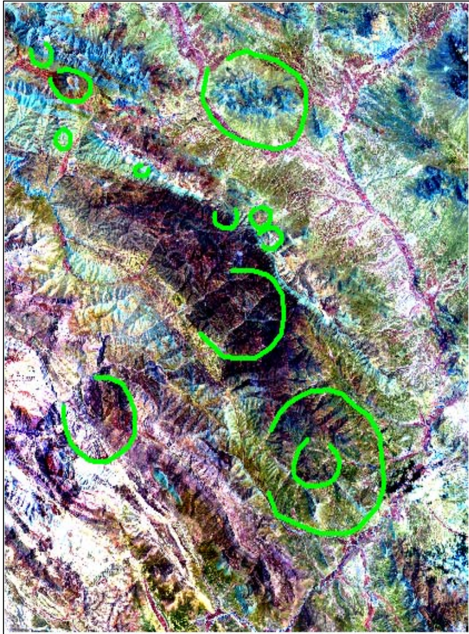
تصویر شماره ۳-۴ - نمایش ساختارهای حلقوی منطقه. ترکیب باندی ۱-۳-۵ سنجنده ETM ماهواره
