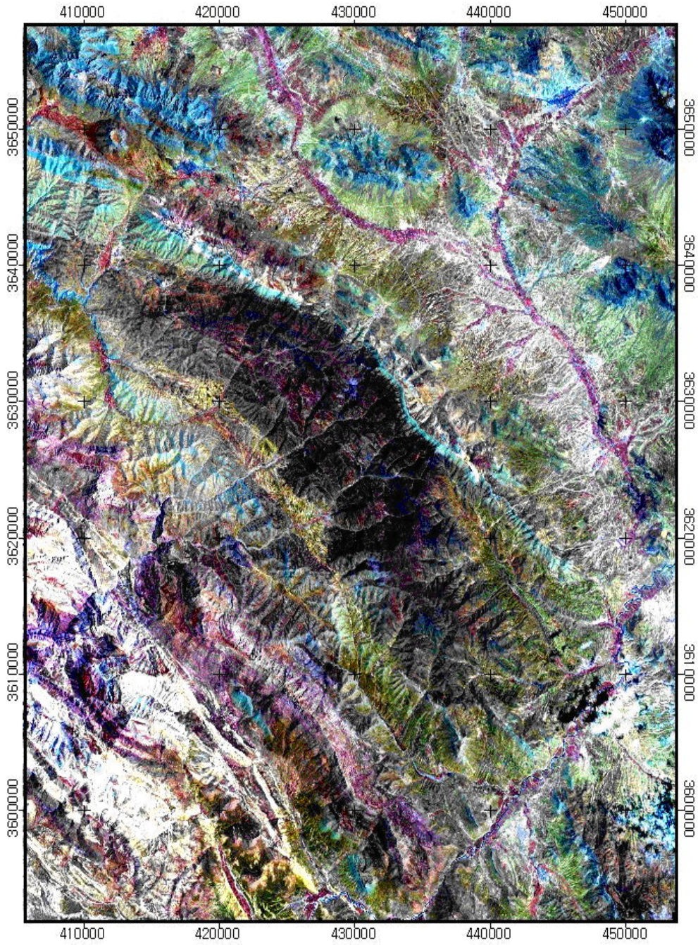
تصویر شماره ۳-۳ - نقشه ماهواره ای ورقه فریدونشهر
