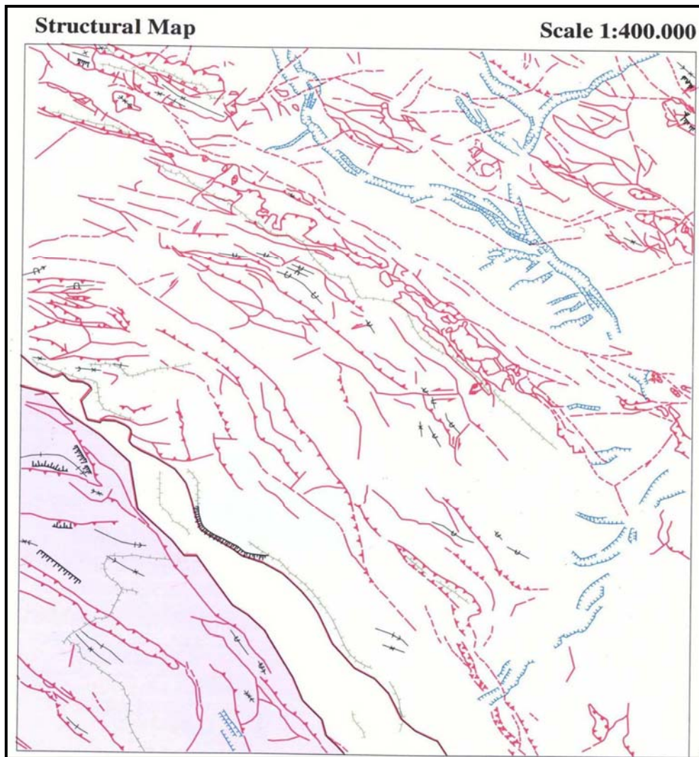
عکس ۲-۳ - نقشه زمین ساخت ورقه ۱:۱۰۰۰۰۰۰ فریدونشهر
