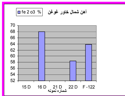
نمودار ۲-۳ - نمودار آهن محدوده شمال خاور غرغن
