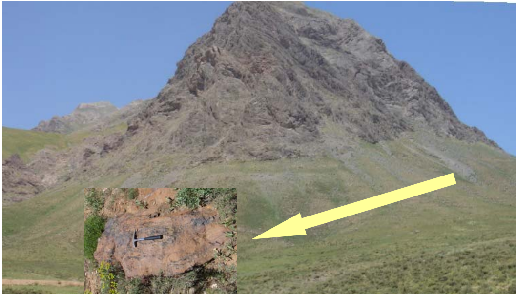
عکس ۳-۶ - محدوده آهن سنگباران (دید به سمت شمال)
