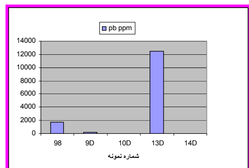
نمودار ۳-۳ - نمودار سرب و روی محدود بل امیر
