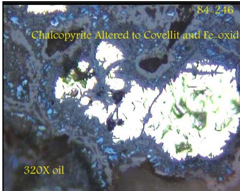
عکس ۴-۴- آلتراسیون کالکوپیریت به کولیت و اکسیدهای آهن
