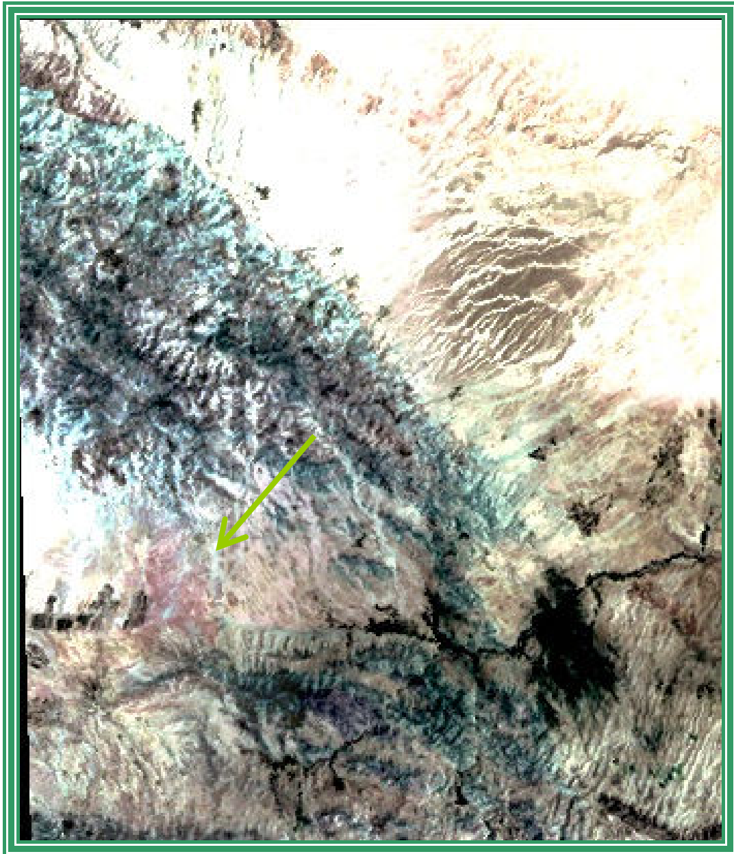
شکل (۳-۱۶) بارزسازی امکان وجود آلتراسیون سیلیسی با استفاده از ترکیب بندی داده های TIR و ASTER
