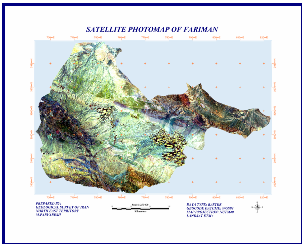
شکل (۳-۶) ترکیب باندی او ۳ و ۵ جهت تفکیک واحدهای زمین شناسی
