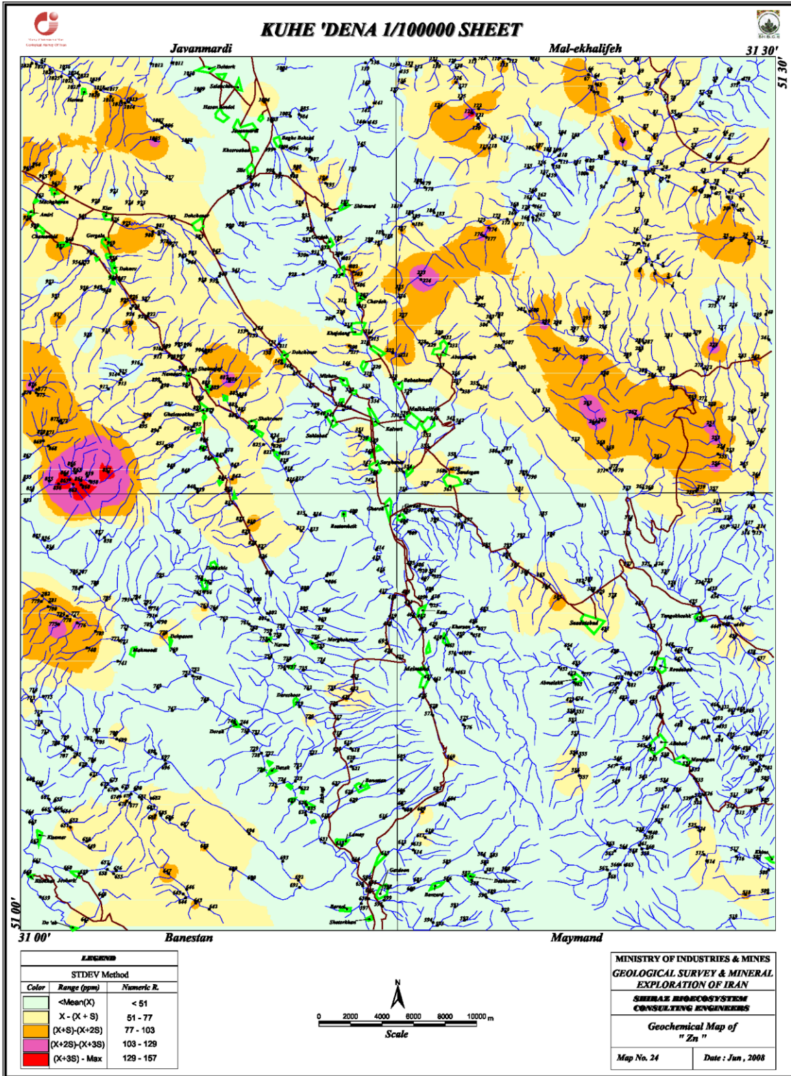
شکل 3-4: نقشه توزیع ژئوشیمیایی عنصر روی در ورقه 1:100000 کوه دنا
