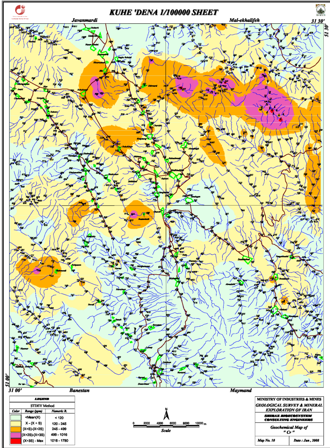
شکل 4-4: نقشه توزیع ژئوشیمیایی عنصر کروم در ورقه 1:100000 کوه دنا
