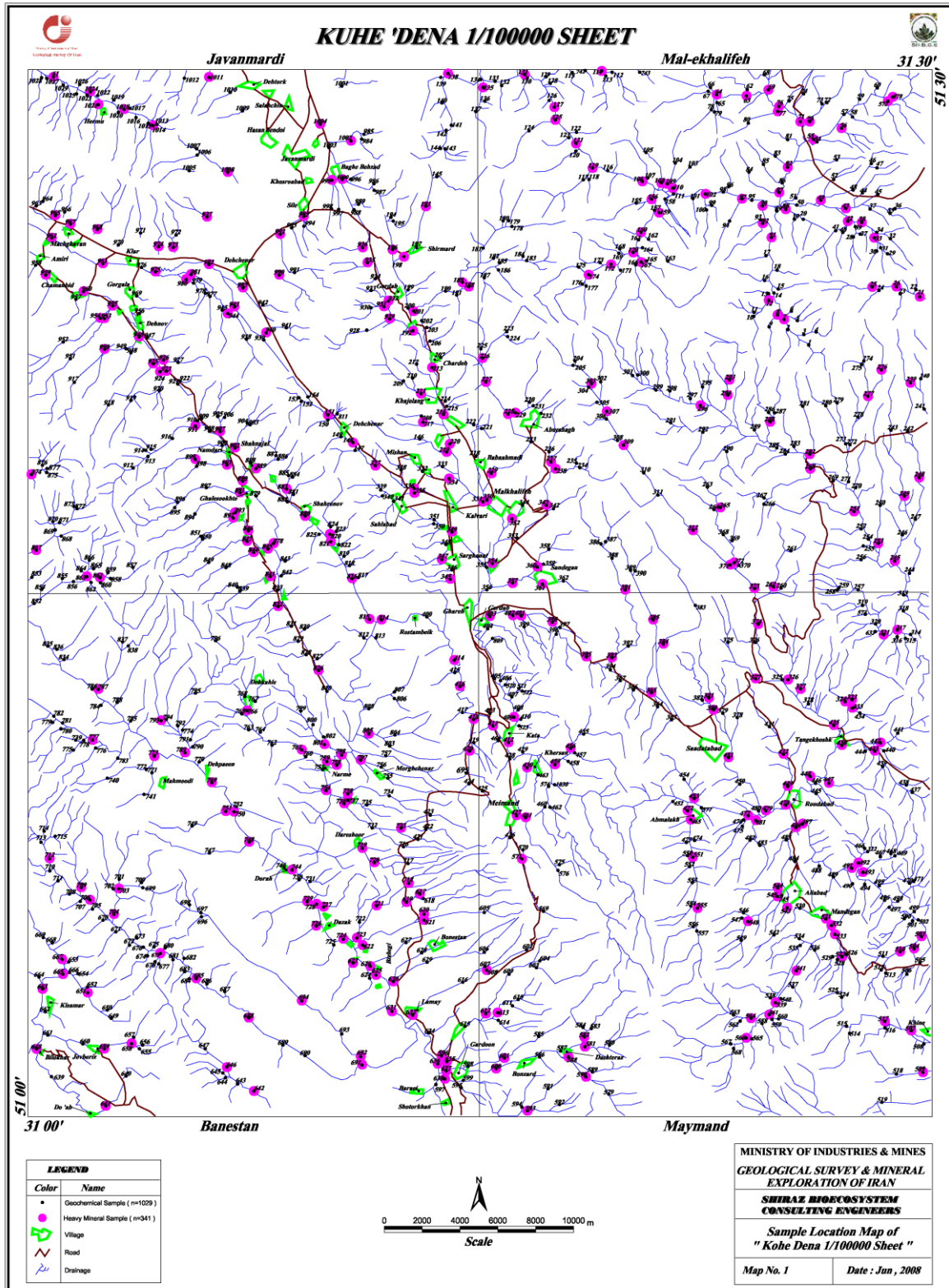
شکل 1-2: موقعیت نمونه های ژئوشیمیایی و کانی سنگین
