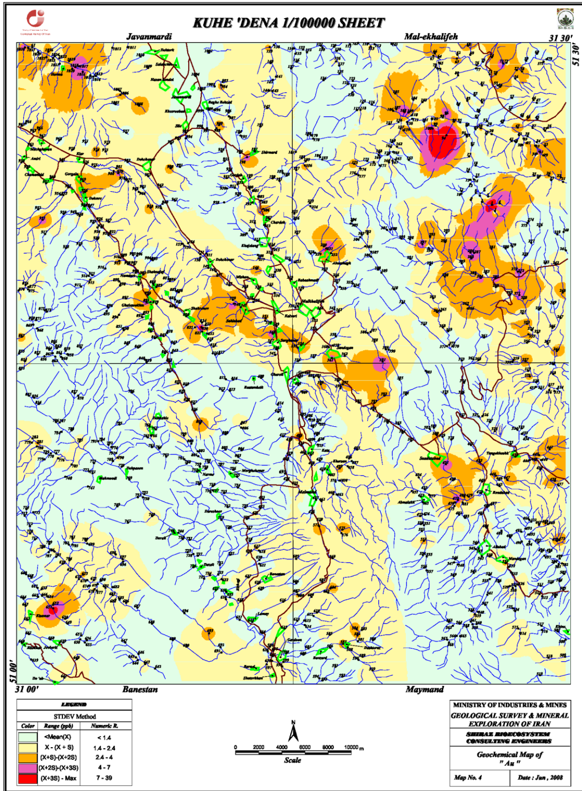
شکل 1-4: نقشه توزیع ژئوشیمیایی عنصر طلا در ورقه 1:100000 کوه دنا
