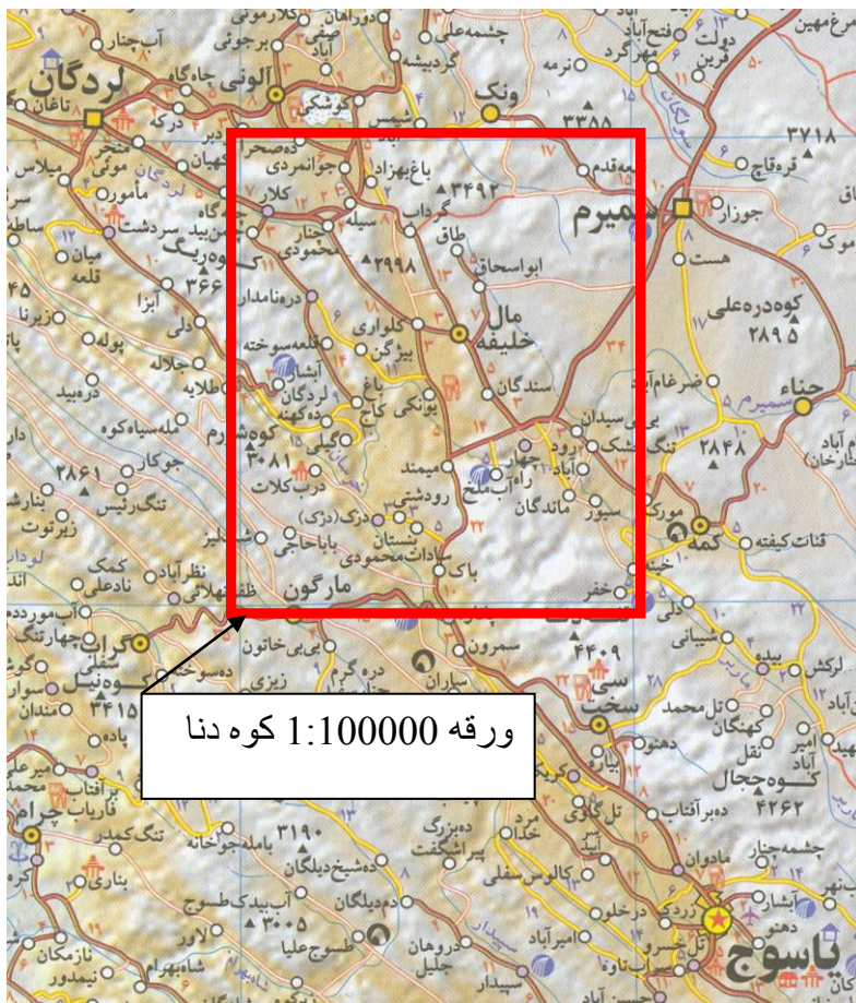
شکل 1-1- موقعیت جغرافیایی و راههای دسترسی به محدوده مورد مطالعه
