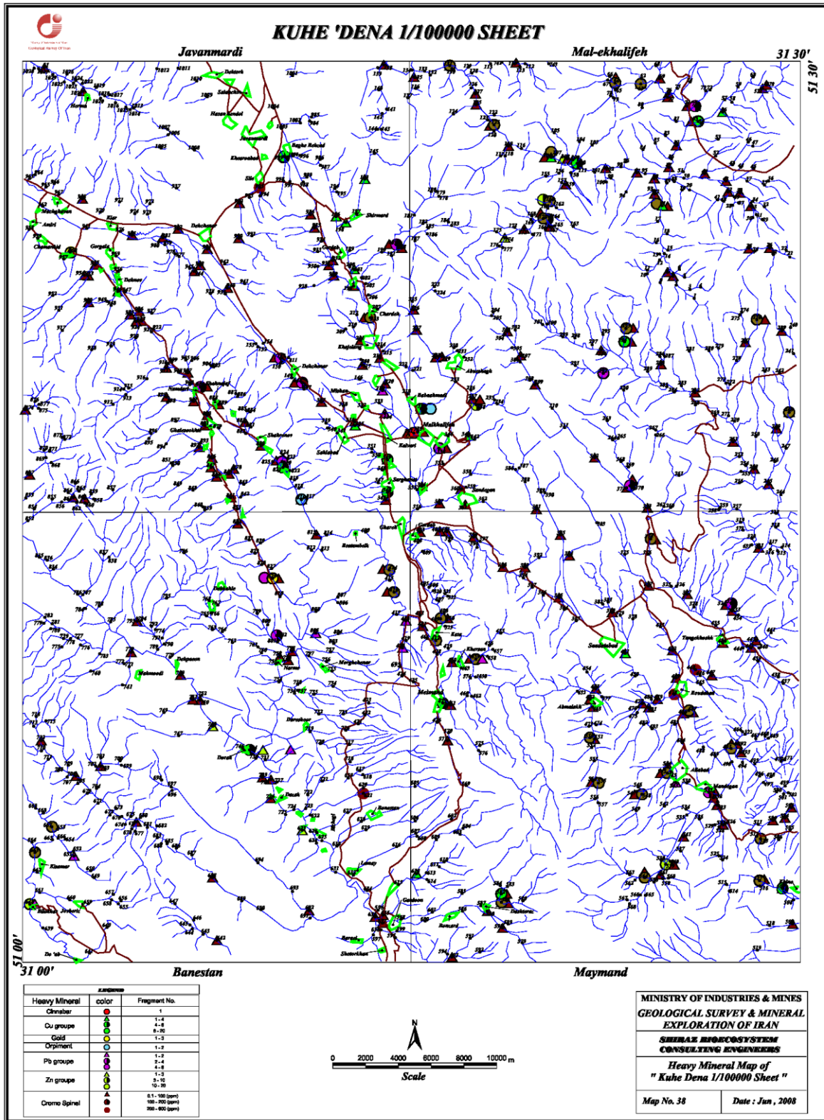
شکل 5-1: نقشه پراکندگی کانی های سنگین در ورقه 1:100000 کوه دنا
