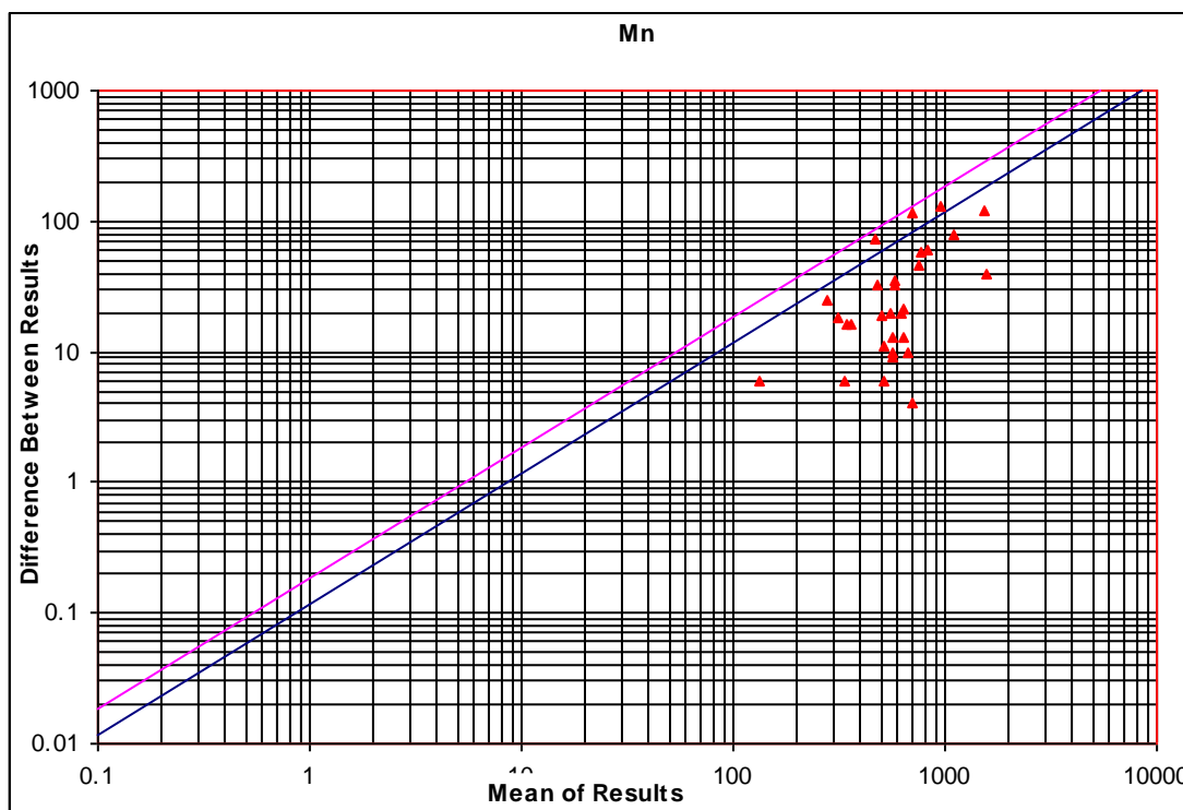
شکل 3-2: نمودارهای کنترل خطا برای عنصر منگنز در ورقه 1:100000 کوه دنا
