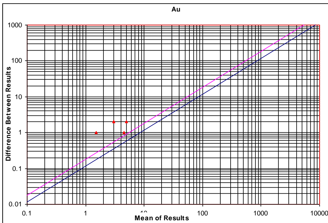
شکل 3-1: نمودارهای کنترل خطا برای عناصر طلا در ورقه 1:100000 کوه دنا
