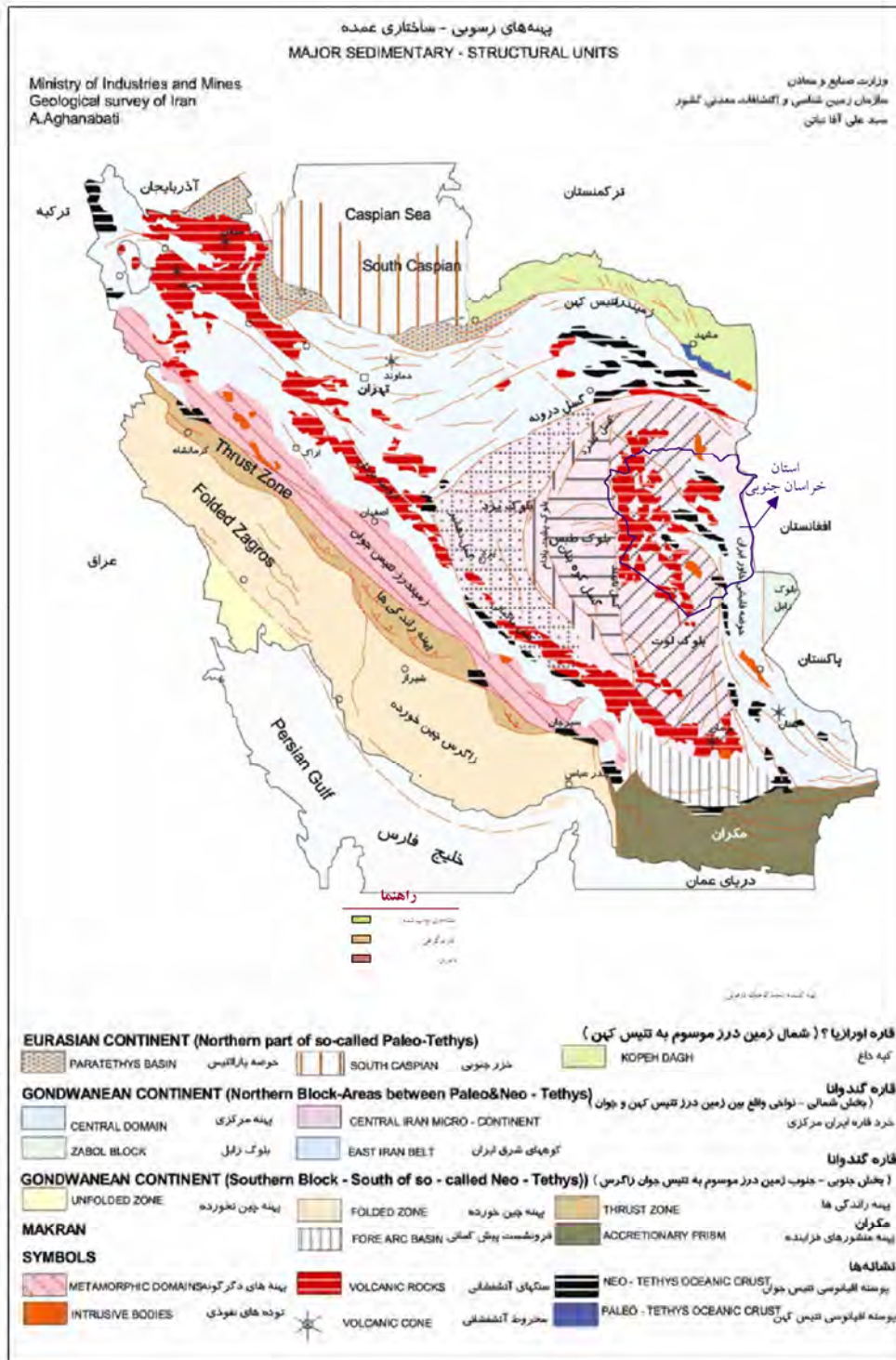
شکل ۳- نقشه پهنه های ساختمانی ایران و موقعیت محدوده مورد
