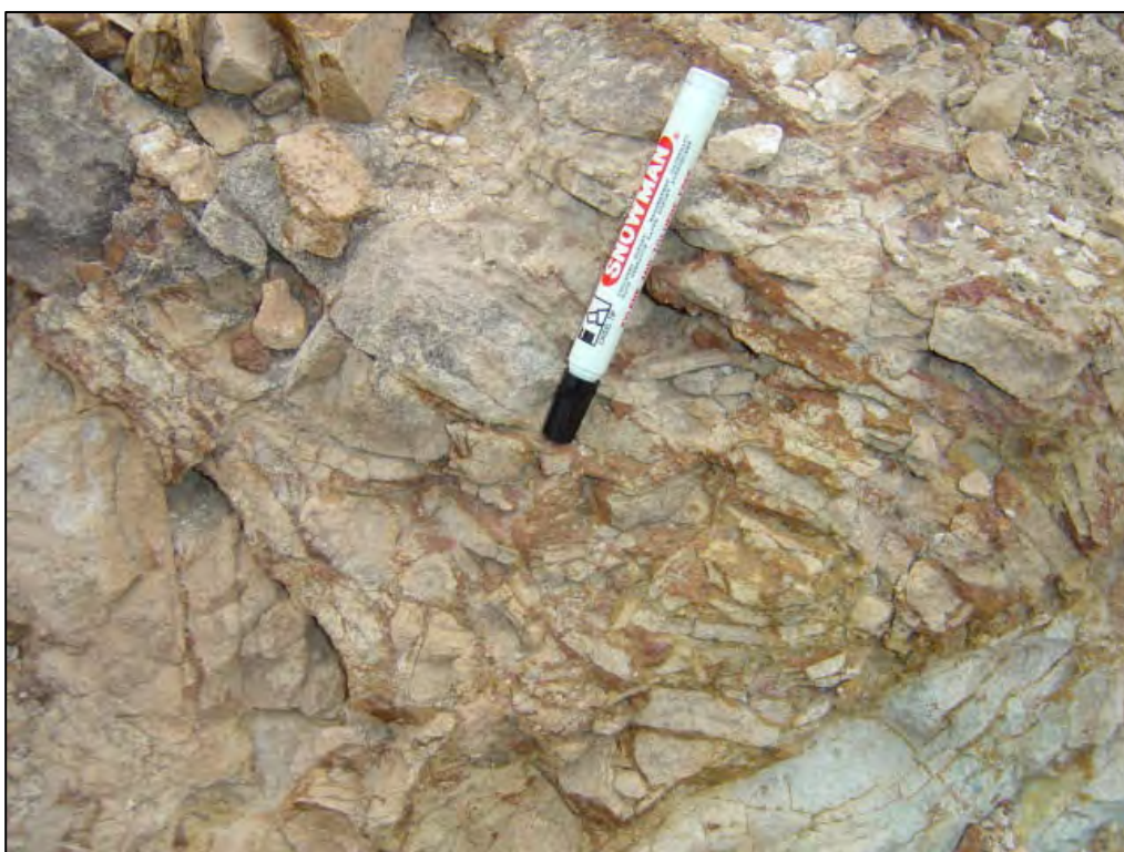
عکس ۶- نمایی نزدیک از تنوره برشی خونیک
