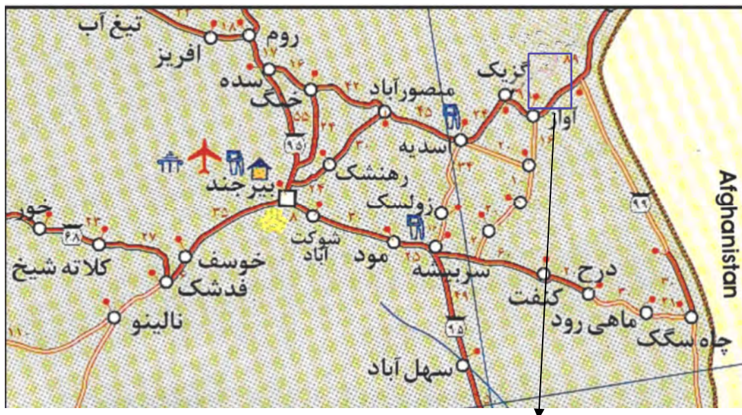
شکل ۹ - موقعیت معادن گرانیت شرق - شمال شرق گزیک
