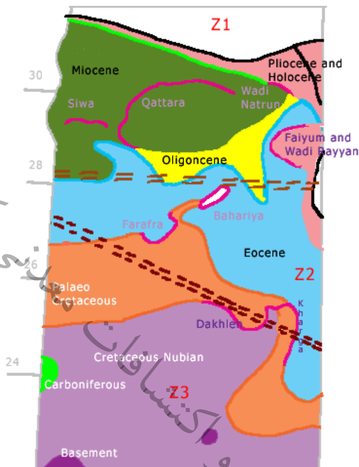
نقشه زمین شناسی غرب کشور مصر
