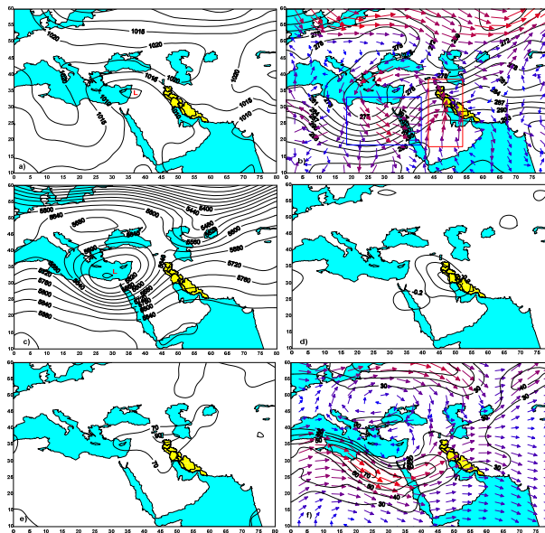
شکل ۵-۱-۳-۵ (a) میدان فشار سطح متوسط دریا (هکتوپاسکال)، (b) میدان باد (متر بر ثانیه) و دما (کلوین) در تراز ۸۵۰ هکتوپاسکال، (c) گرته ارتفاع تراز ۵۰۰ هکتوپاسکال (ژئوپتانسیل متر)، (d) مقادیر منفی مولفه قائم سرعت باد (پاسکال بر ثانیه)، (e) رطوبت نسبی تراز ۷۰۰ هکتوپاسکال (درصد) و (f) میدان باد تراز ۲۰۰ هکتوپاسکال (متر بر ثانیه) در ساعت ۰۰۰۰ گرینویچ روز ۳۱ مارس ۲۰۱۹.
