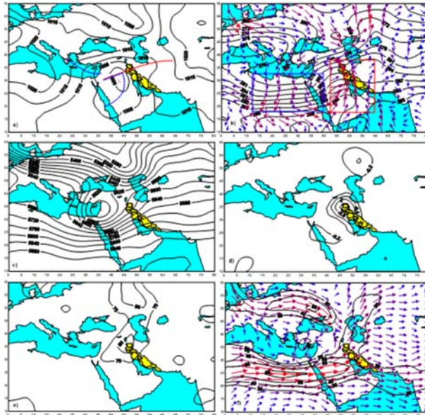
شکل ۵-۱-۲-۵ (a) میدان فشار سطح متوسط دریا (هکتوپاسکال)، (b) میدان باد (متر بر ثانیه) و دما (کلوین) در تراز ۸۵۰ هکتوپاسکال، (c) گرته ارتفاع تراز ۵۰۰ هکتوپاسکال (ژئوپتانسیل متر)، (d) مقادیر منفی مولفه قائم سرعت باد (پاسکال بر ثانیه)، (e) رطوبت نسبی تراز ۷۰۰ هکتوپاسکال (درصد) و (f) میدان باد تراز ۲۰۰ هکتوپاسکال (متر بر ثانیه) در ساعت ۰۰۰۰ گرینویچ روز ۲۵ مارس ۲۰۱۹.
