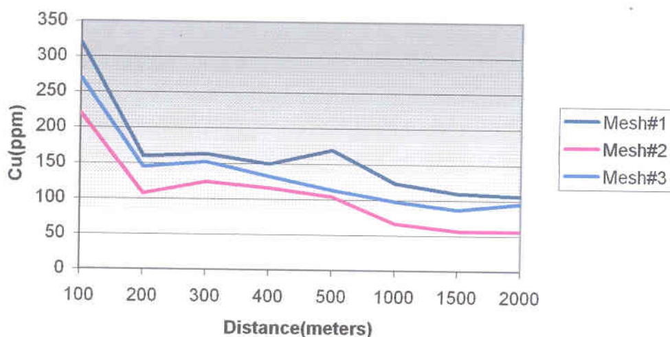
شکل شماره ۲-۲: دیاگرام شماتیک عیار - فاصله برای دانه بندیهای مختلف
