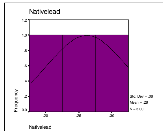
شکل ۳-۱: هیستوگرام فراوانی کانیهای سنگین در برکه ۱:۲۵۰۰۰ نرده ۲
