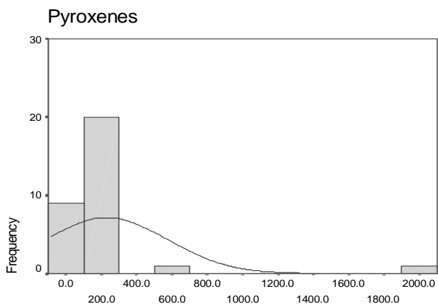
Pyroxenes
