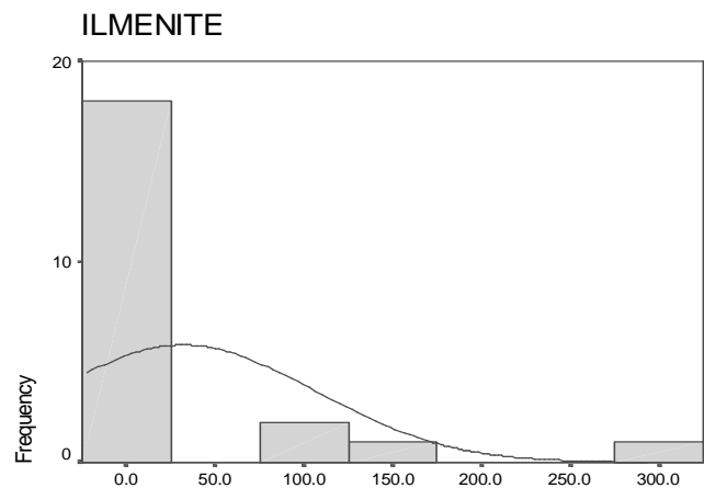
ILMENITE
