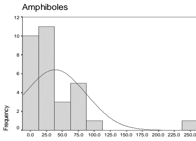
Amphiboles
