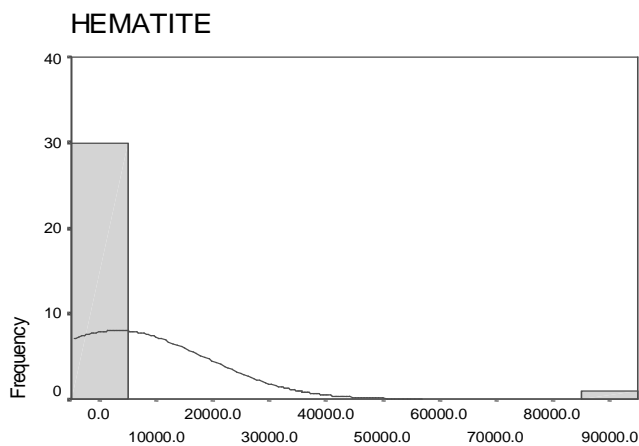
HEMATITE
