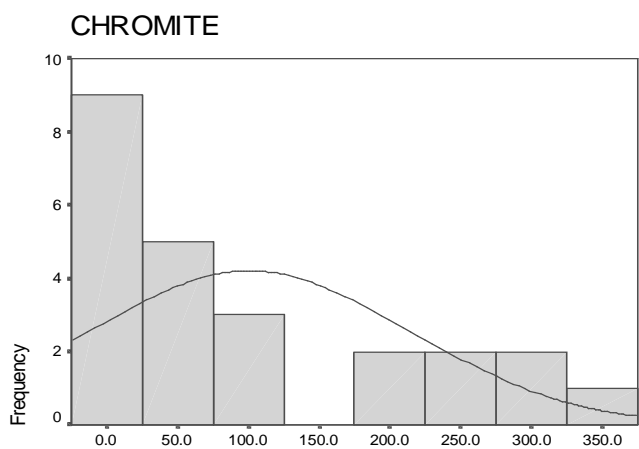
CHROMITE
