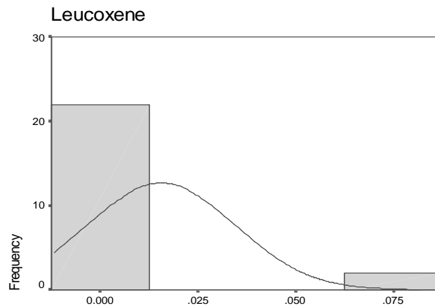
Leucoxene
