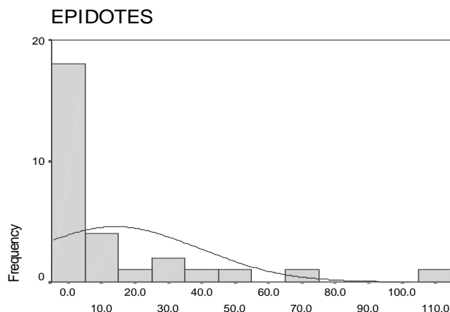
EPIDOTES
