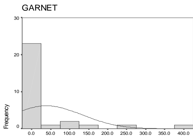
GARNET
