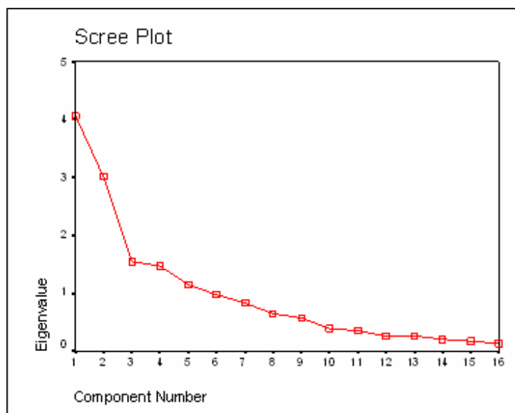
شکل (۳-۵): نمودار صخره ای برای تعیین بهینه تعداد عاملها
