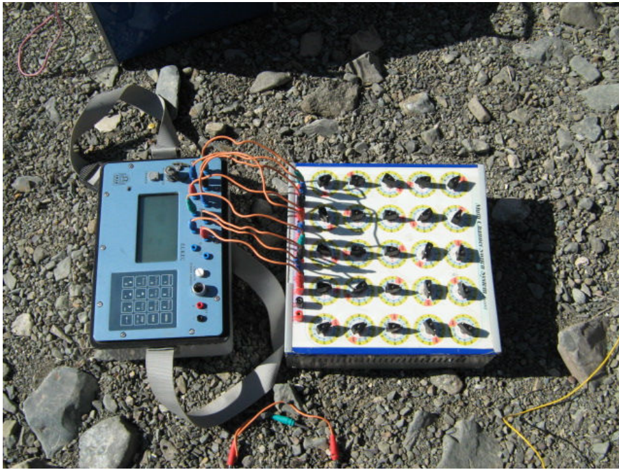
تصویر شماره ۱۳- گیرنده (رسیور) ELREC-10 ساخت شرکت IRIS فرانسه به همراه سویچ باکس ساخت سازمان زمین شناسی کشور (گروه ژئوفیزیک)
