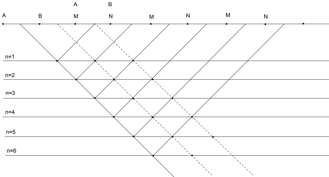
شکل ۶- آرایش دوقطبی-دوقطبی
