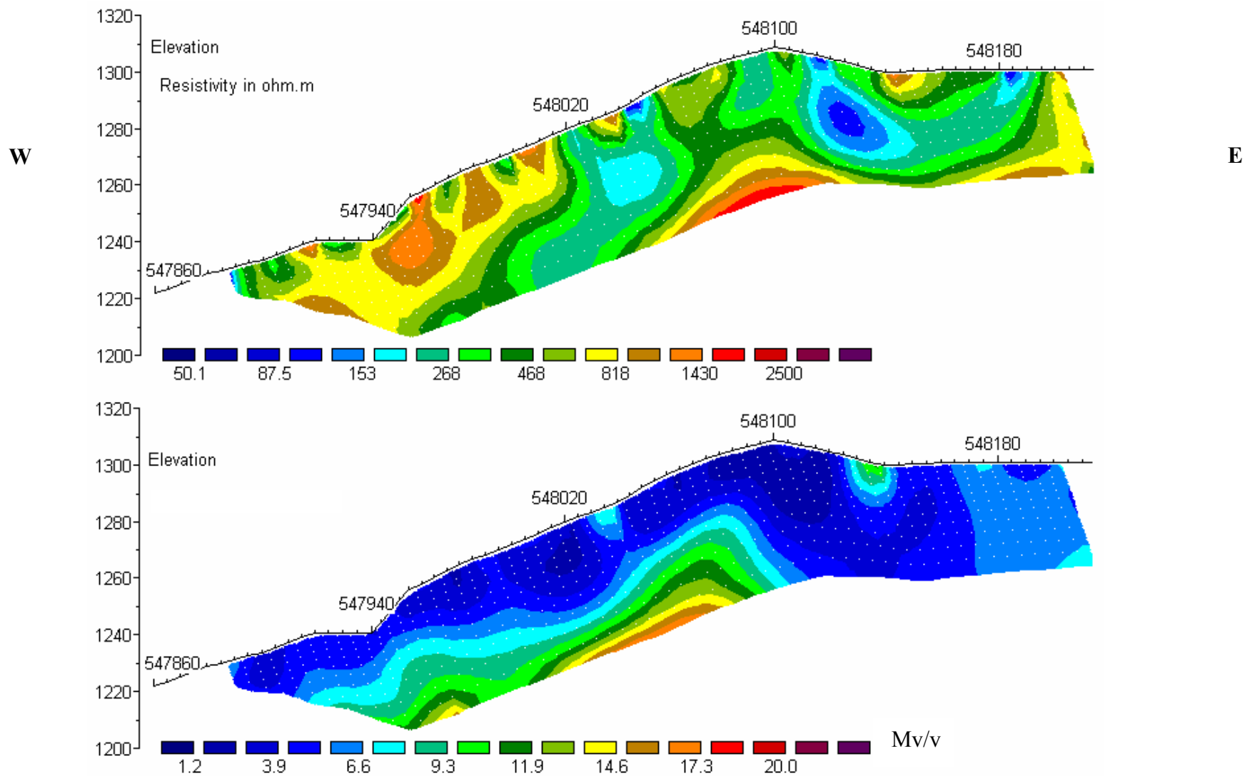
نقشه شماره ۳۱- مدل مقاومت ویژه و پلاریزاسیون القایی بر روی پروفیل شماره ۱۰ با UTM ۳۱۵۴۲۰۰ شمالی
