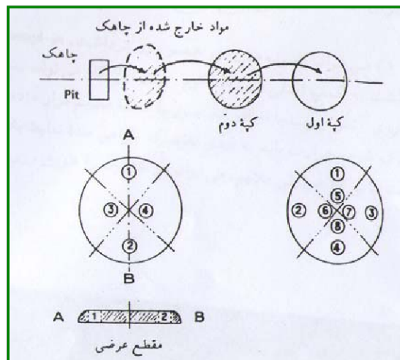
شکل ۳-۴ : برداشت نمونه از شن‌های خارج شده و مخلوط شده از چاهک‌های اکتشافی.
