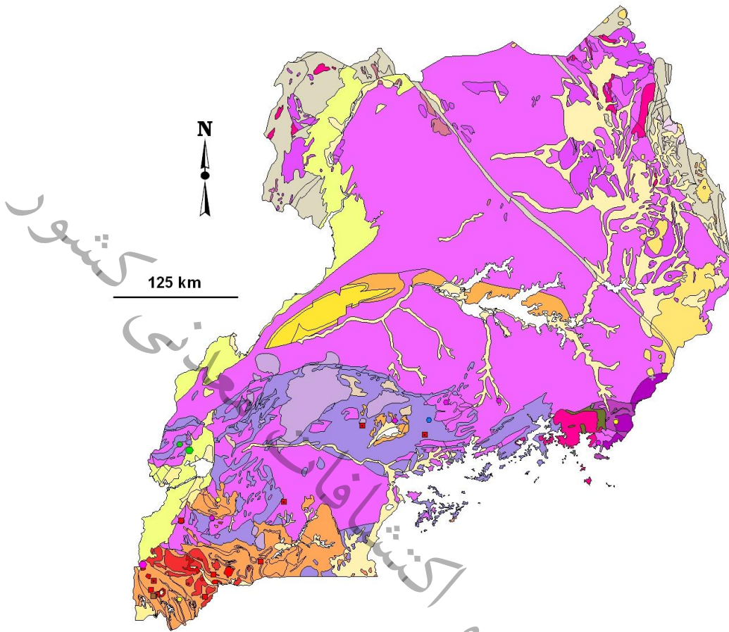
نقشه زمین شناسی کشور اوگاندا
